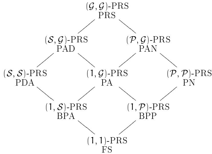
Fig. 2. The PRS-Hierarchy
